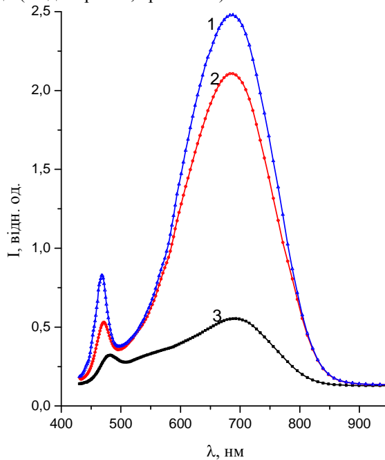
Рис. 6. Спектри люмінесценції НК CdS, виміряні за температур 300 (1), 150 (2) та 77 К (3).
