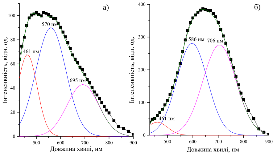
Рис. 3: Апроксимація кривими Гауса спектрів люмінесценції зразків, отриманих при мольному співвідношенні вихідних компонент CdNO 3 /Na 2 S : 2/1(зразок 2) (а); 1/4 (зразок 3) (б).
