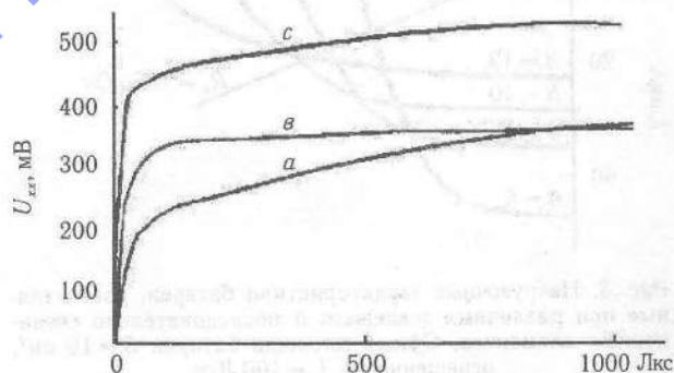
Рис. 2. Зависимость U_{\text{ХХ}} от освещенности для фотоэлементов:
