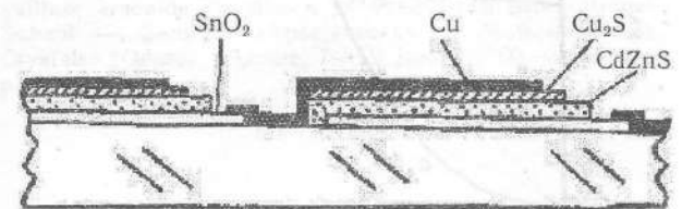
Рис. 5. Схематическое изображение фрагмента фотоэлектрической батареи
