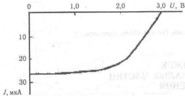
Рис. 6. Экспериментальная нагрузочная характеристика фотоэлектрической батареи из 10 последовательно соединенных элементов. Общая площадь P = 10 \text{ см}^2 , освещенность L = 100 \text{ Лкс} .
