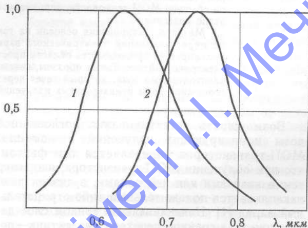
Рис. 2. Спектральное распределение фотолюминесценции монокристалла CdS (1) и нанокристаллов CdS в желатиновой матрице (2), измеренные при 300 К
